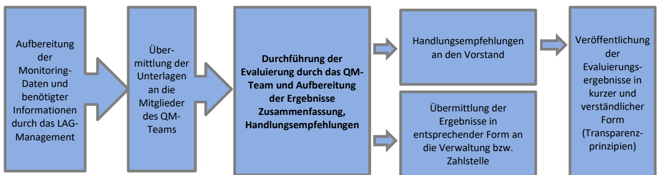
Abbildung 13: Ablauf Qualitätsmanagement
